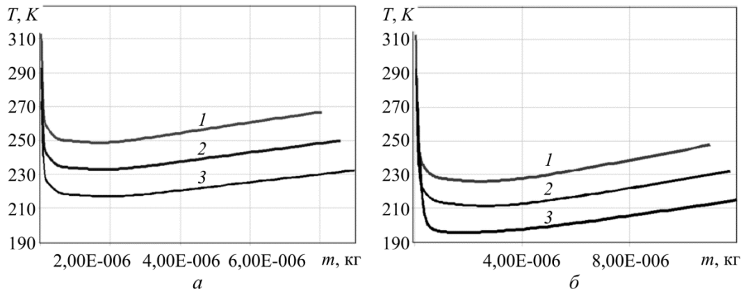
Рис. 8. Изменение температуры газа внутри оболочки в зависимости от его массы в начале процесса развертывания: a – воздух; б – гелий. Начальная температура и температура вдуваемого газа одинакова. 1 – 273К; 2 – 293К; 3 – 303К
