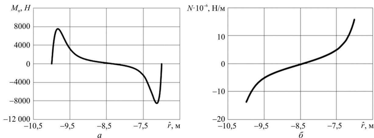
Рис. 2. Изменение изгибающего момента M_\varphi ( а ) и окружного усилия N ( б )
