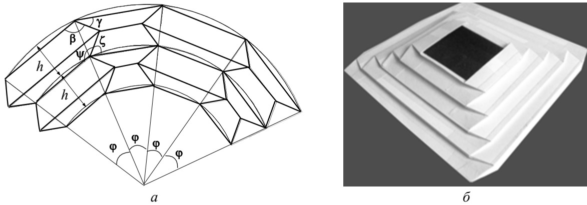
Рис. 6. Развертка двухполосной конической оболочки с нанесенными линиями сгиба (а), оригами упакованной оболочки (б) Fig. 6. Deployment of a dual-band cone-shaped shell with fold lines (а), origami of the packed shell (б)
