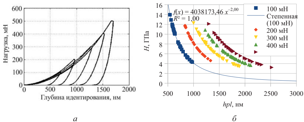
Рис. 3. Типичные кривые индентирования композита по первой схеме нагружения ( a ); зависимость значений нанотвердости H от глубины отпечатка hpl для различных значений максимальных приложенных усилий ( б )
