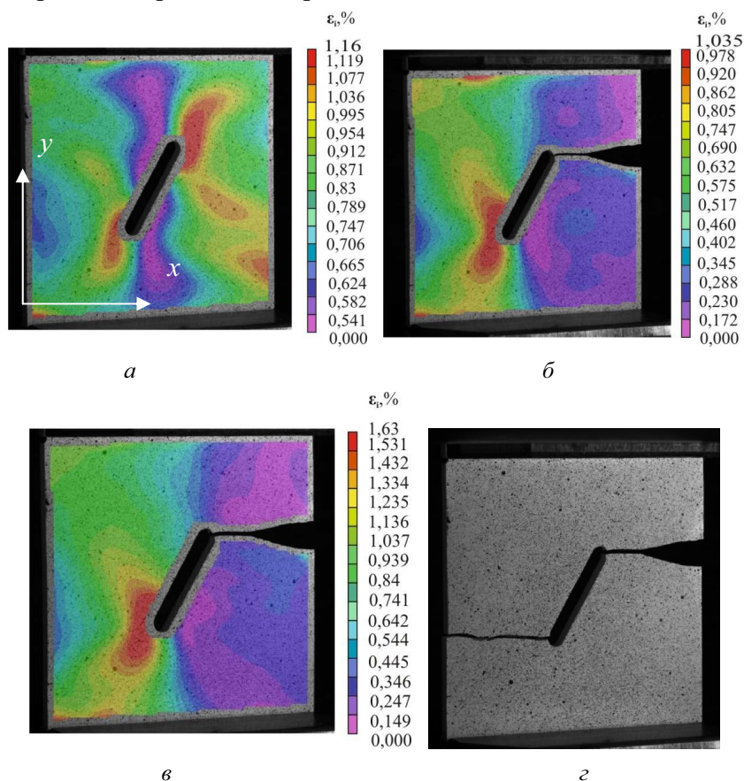
Рис. 6. Поля интенсивности деформаций \epsilon на поверхности образца, где ось выреза составила со стороной пластины 60^\circ при нагрузке P_1 = 2,837 кН (а); P_2 = 1,243 кН (б); P_3 = 1,713 кН (в); фото разрушенного образца (г)
