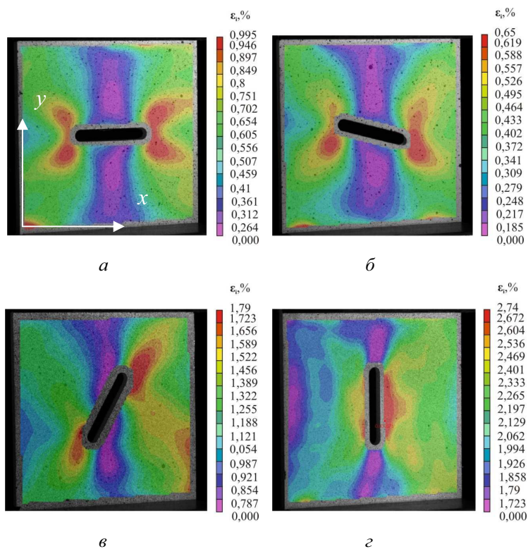
Рис. 4. Поля интенсивности деформаций \epsilon_i на поверхности пластин, ось выреза составляла со стороной пластины 0^\circ (а), 15^\circ (б), 60^\circ (в), 90^\circ (г)
