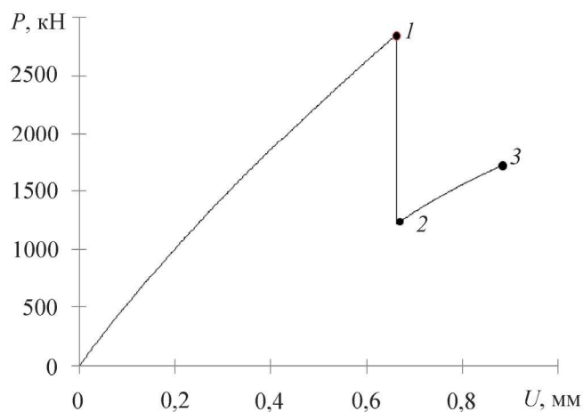
Рис. 5. Диаграмма нагружения для образца, где ось выреза составляла со стороной пластины 60^\circ
