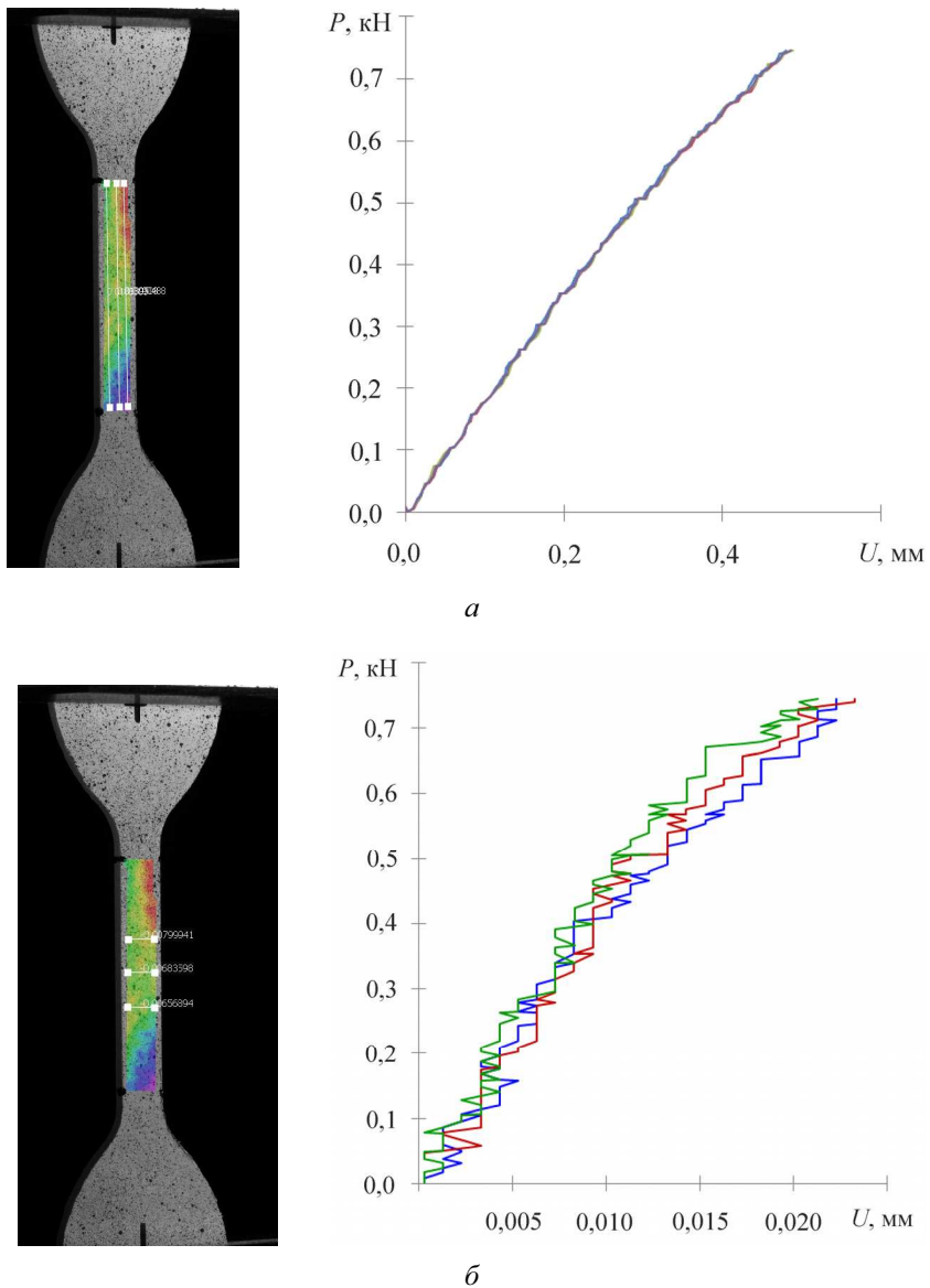
Рис. 1. Регистрация продольной (а) и поперечной деформации (б) в процессе нагружения с использованием дополнительного модуля программного обеспечения оптической системы «виртуальный экстензометр»
