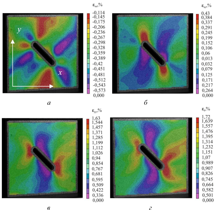
Рис. 3. Поля поперечных \epsilon_{xx} (а), сдвиговых \epsilon_{xy} (б); продольных деформаций \epsilon_{yy} (в) и интенсивности деформаций \epsilon_i (г) на поверхности пластины ( \alpha=45^\circ ) при нагрузке 3,731 кН (см. также с. 191)
