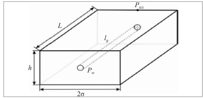
Рис. 3. Горизонтальная скважина в прямоугольном нефтяном пласте
