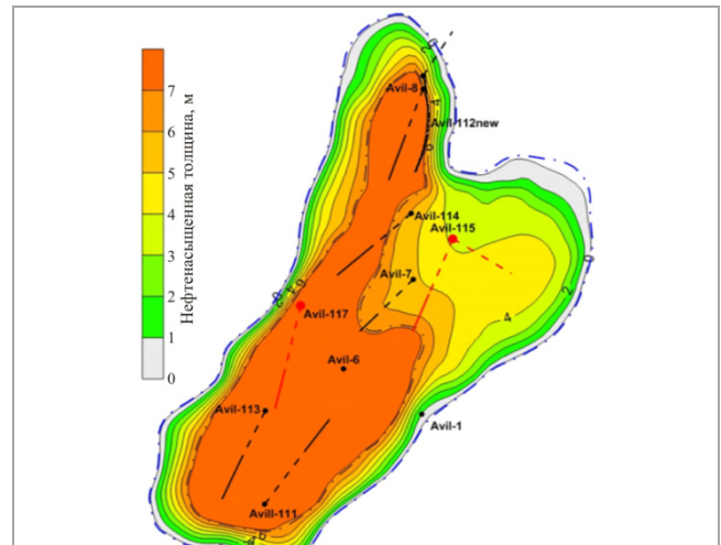
Рис. 5. Авиловское газонефтяное месторождение
