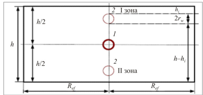
Рис. 2. Асимметричное расположение ствола горизонтальной скважины по отношению к кровле и подошве полосовидного пласта
