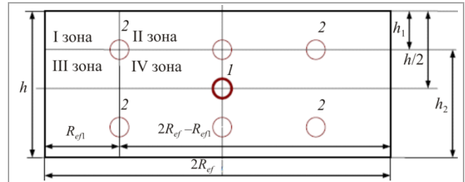
Рис. 4. Схема условного расположения горизонтальной скважины в пласте: 1 – симметричное; 2 – асимметричное
