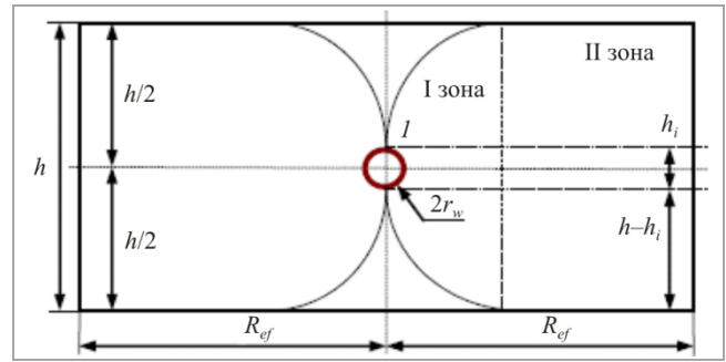
Рис. 1. Схема расположения симметричного ствола горизонтальной скважины по толщине пласта
