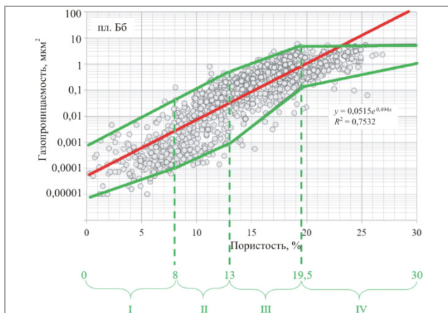
Рис. 1. Зависимость проницаемости от пористости по данным исследования керна
