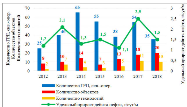
Рис. 2. Динамика количества выполненных ГРП, количества объектов применения, количества технологий ГРП и удельного прироста дебита нефти после ГРП на месторождениях Республики Коми и Ненецкого АО с 2012 по 2018 г.
