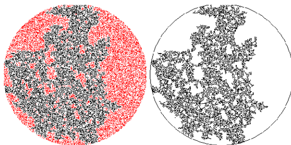
Рис. 5. Пример кластера: а – скопление бактерий; б – наибольший кластер
