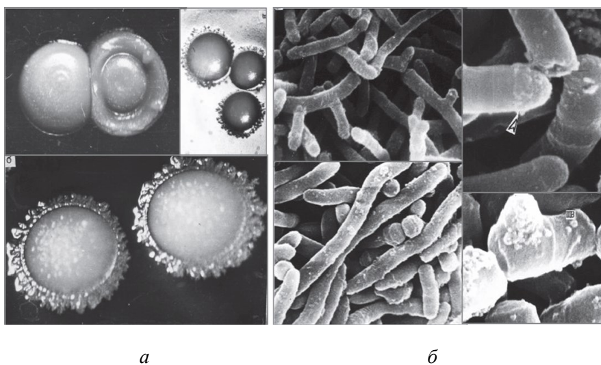
Рис. 1. Колонии (а) и клетки (б) родококков [2]
