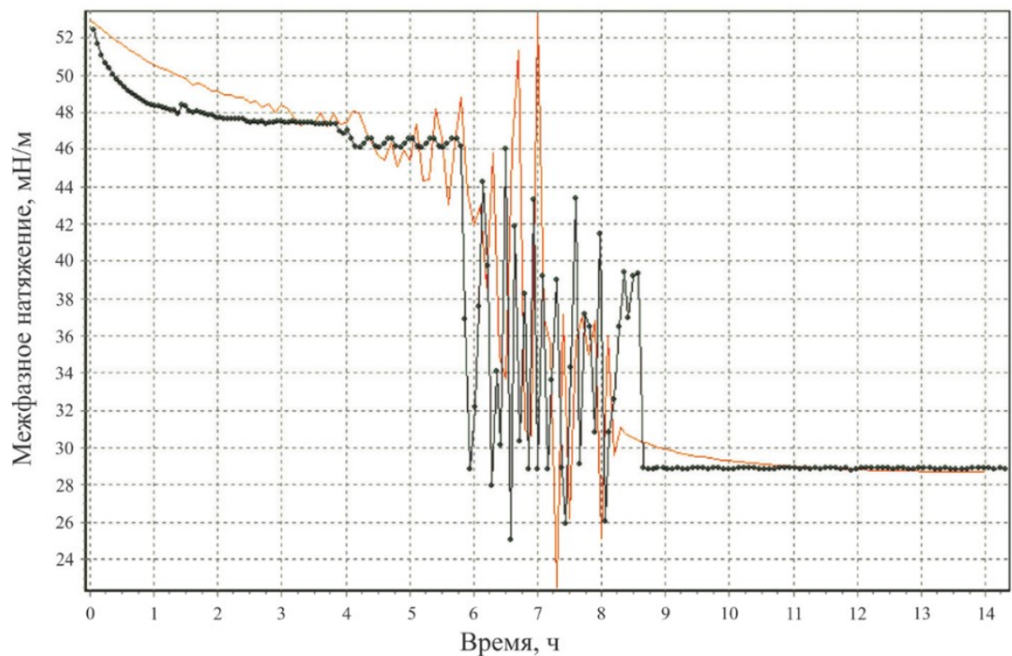
Рис. 4. Экспериментальная зависимость \sigma(t) ( OP_{600nm} = 0,75 ) и соответствующая теоретическая зависимость, не учитывающая ( a ) и учитывающая ( б ) случайные вариации
