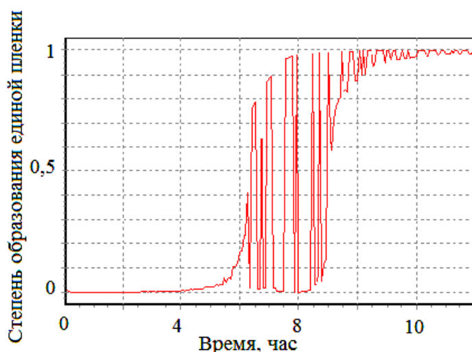
Рис. 6. Зависимость s(t) в модели формирования и разрушения кластеров
