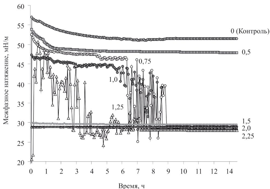
Рис. 2. Динамика межфазного натяжения суспензии клеток R. ruber ИЭГМ 231 в системе вода – n -гексадекан. Значения OP_{600nm} клеточных суспензий: 0; 0,5; 0,75; 1,0; 1,25; 1,5; 2,0; 2,25
