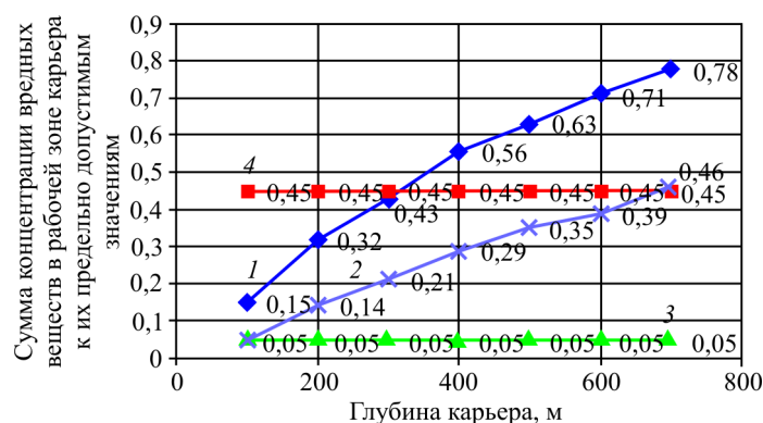
Рис. 1. Изменение суммы концентрации вредных веществ в рабочей зоне карьера к их предельно допустимым значениям для различных видов транспортных машин при изменении глубины карьера [9]: 1 – дизельный автомобильный транспорт; 2 – дизель-троллейвозный транспорт; 3 – конвейерный транспорт; 4 – максимальная допустимая концентрация
