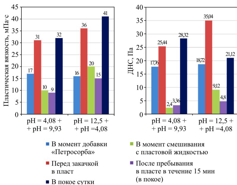
Рис. 5. Изменение показателей пластической вязкости и ДНС 2%-ного бурового раствора (pH = 4,08 и pH = 12,5) с добавлением «Петросорба»
