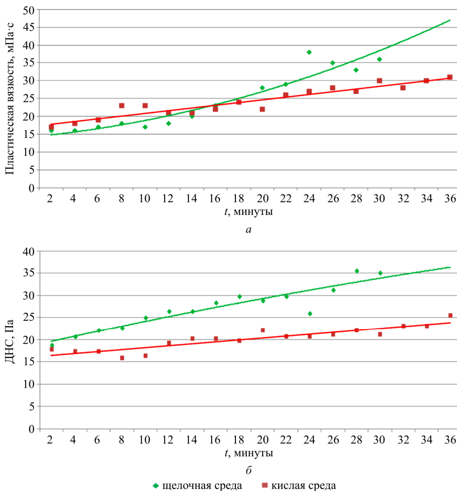
Рис. 4. Зависимость: a – пластической вязкости; б – ДНС от времени бурового раствора различного pH с добавлением «Петросорба»
