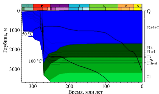
Рис. 3. Комплексная модель погружения, прогрева и нефтегенерации аллохтона Вуктыльского надвига по данным параметрической скв. Вуктыльская-58. Условные обозначения см. на рис. 2
