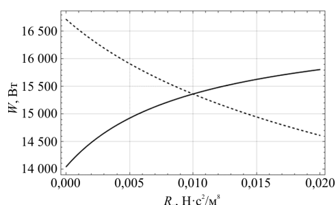
Рис. 7. Мощности, затрачиваемые на проветривание рудничной вентиляционной сети естественной тягой, для режима проветривания по часовой стрелке (..... — скиповый ствол является вентиляционным) и режима проветривания против часовой стрелки (— — скиповый ствол является воздухоподающим)
