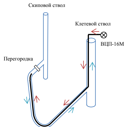
Рис. 1. Схема расчетной модели
