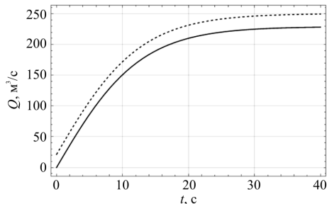
Рис. 3. Изменение расходов воздуха в клетевом (.....) и скиповом (—) стволах с течением времени
