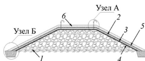
Рис. 1. Конструкция консервации терриконика: 1 – тело терриконика; 2 – гидроизоляционный слой; 3 – газодренажный слой; 4 – разделительный геотекстильный материал; 5 – водно-дренажный слой; 6 – защитный слой грунта
