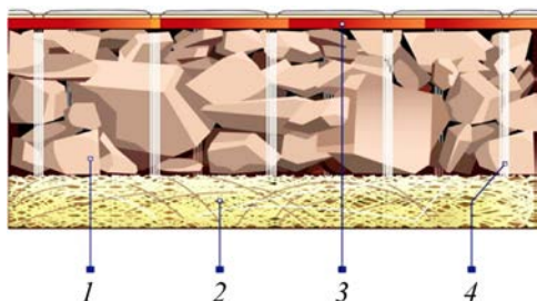
Рис. 4. Структура бентомата: 1 – гранулы бентонита; 2 – нетканое геотекстильное полотно; 3 – тканое геотекстильное полотно; 4 – иглопробивные волокна
