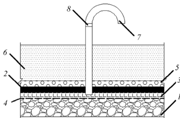
Рис. 2. Узел А устройства вытяжной трубы; 1 – тело терриконики; 2 – гидроизоляционный слой; 3 – газодренажный слой; 4 – разделительный геотекстильный материал; 5 – водно-дренажный слой; 6 – защитный слой грунта; 7 – вытяжная труба; 8 – обратный клапан
