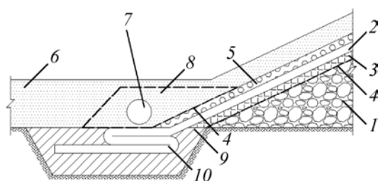
Рис. 3. Узел Б примыкания гидроизоляционного материала к откосам терриконика: 1 – тело терриконика; 2 – гидроизоляционный слой; 3 – газодренажный слой; 4 – разделительный геотекстильный материал; 5 – водно-дренажный слой; 6 – защитный слой грунта; 7 – дренажная труба; 8 – дренажная призма; 9 – пластичный грунт в штрабе; 10 – компенсирующая складка
