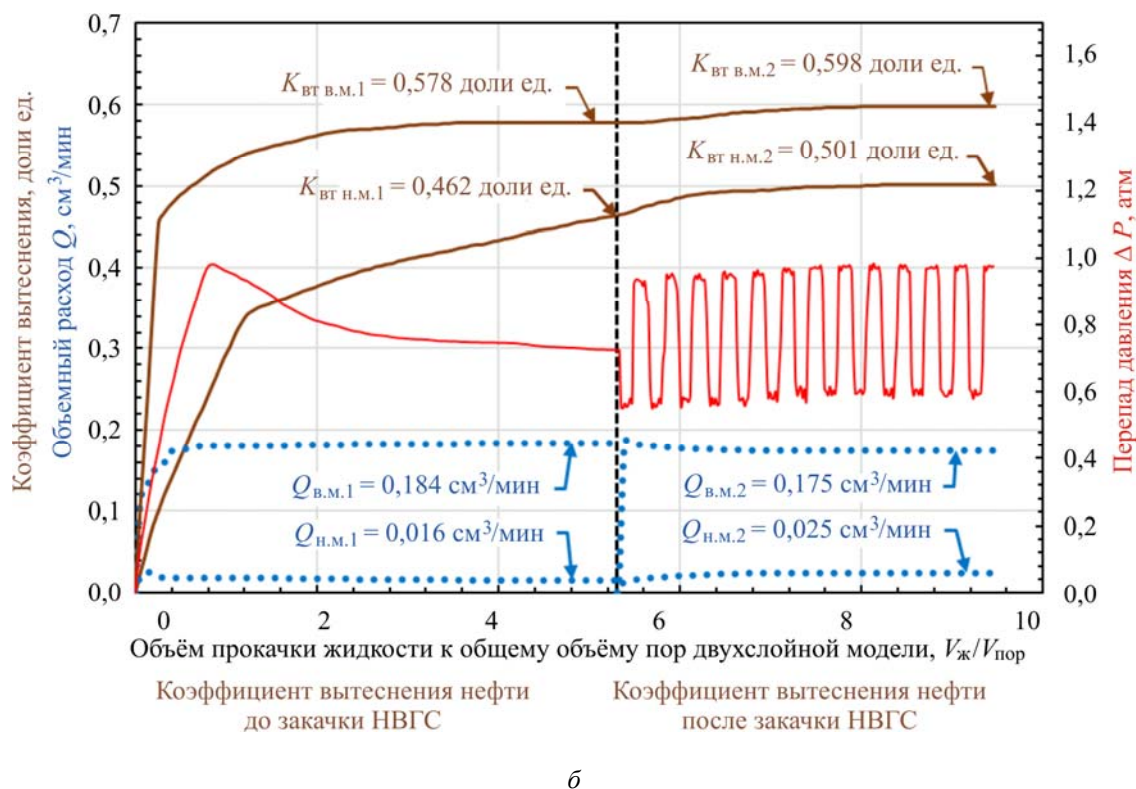
Рис. 2. Динамика основных показателей для двухслойной модели 1 (а) и модели 2 (б) при закачке НВГС: в.п. – высокопроницаемая модель; н.м. – низкопроницаемая модель; нижние индексы 1 и 2 – до воздействия и после воздействия соответственно
