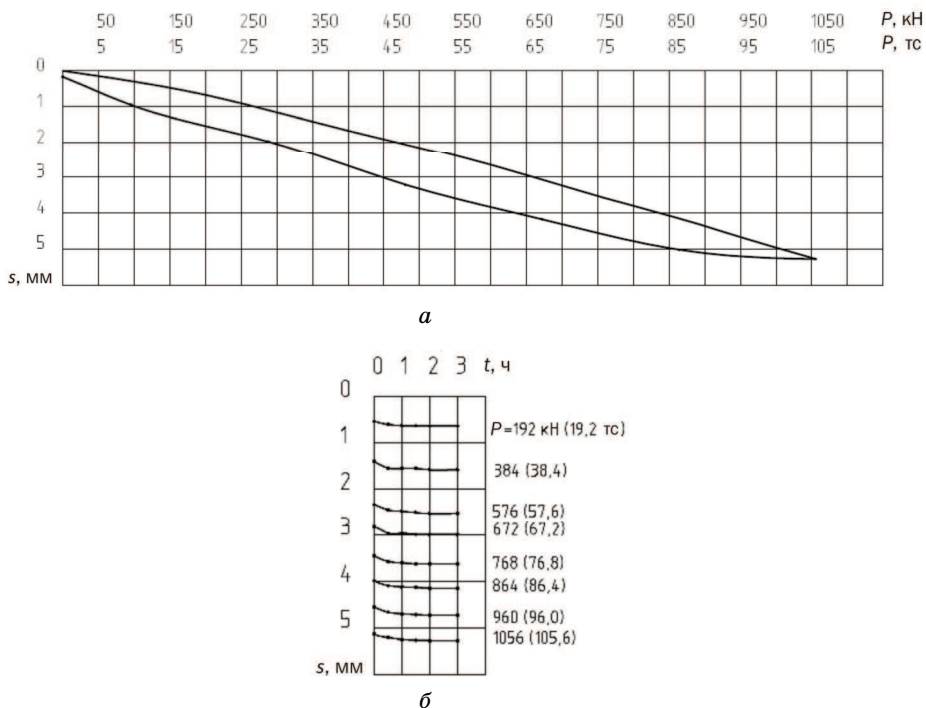
Рис. 3. Результаты испытания сваи статической нагрузкой: а – зависимость осадки сваи s от нагрузки P ; б – изменение осадки сваи s во времени (по ступеням нагружения)
