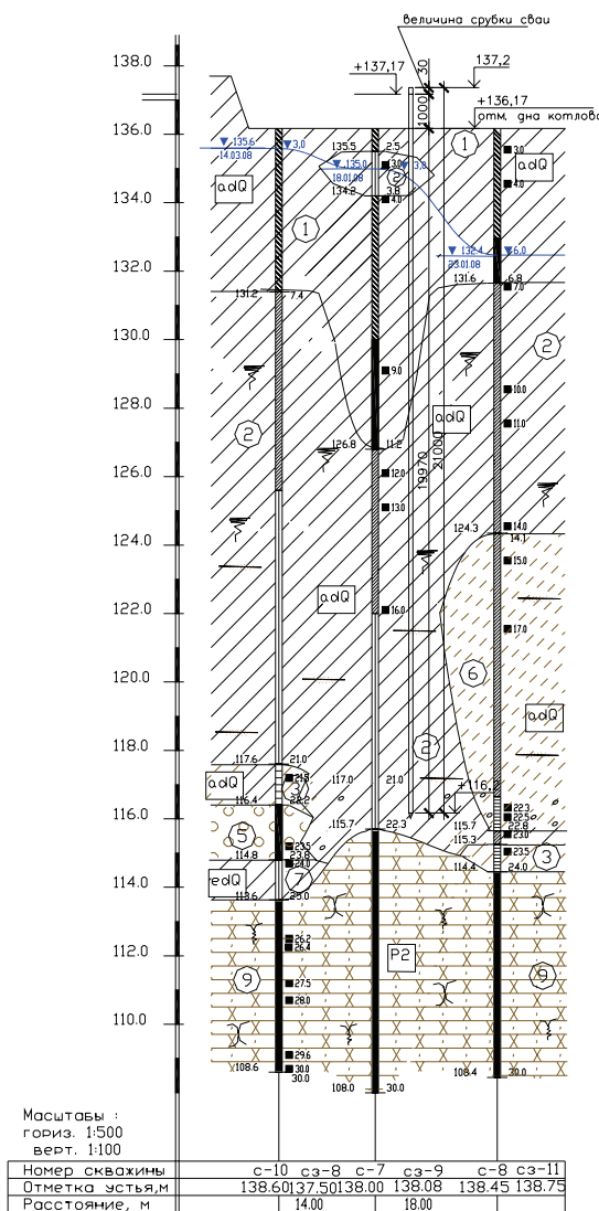
Рис. 1. Инженерно-геологический разрез площадки:
